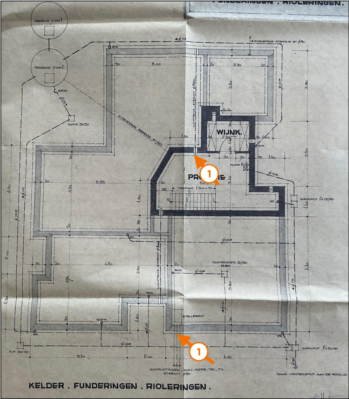
Legende van plan 1.3: Kelder
